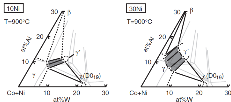
Figura 1. Seções isotérmicas a 900 °C do sistema quaternário Co-Ni-Al-W. Retirado e adaptado de (SHINAGAWA et al., 2008).
